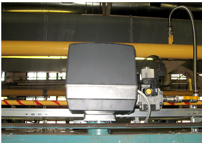
Система нагрева ГАСОМАР с горелками Weishaupt, пламя направлено вертикально вниз
